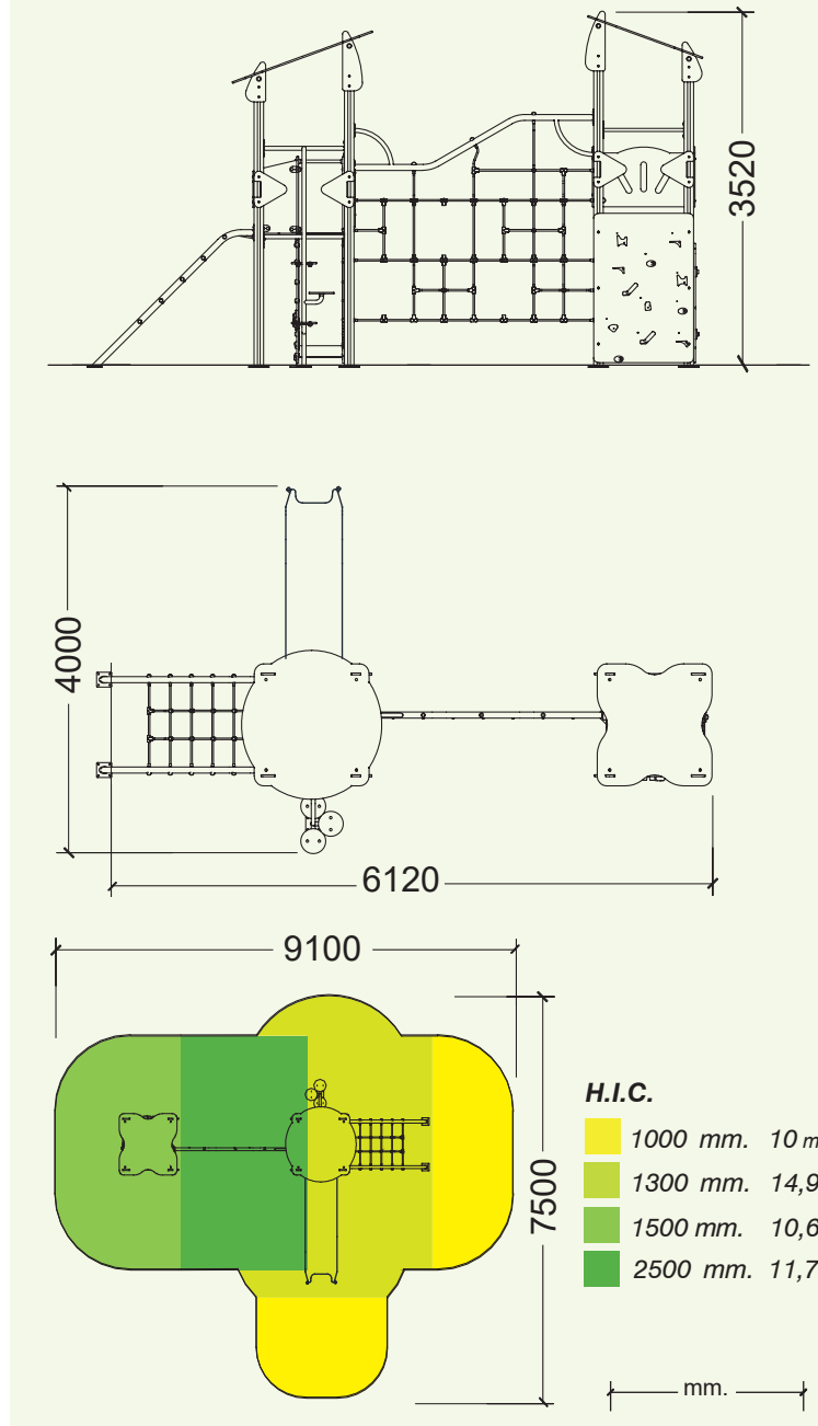
COMPLEJO DE TREPA 2 TORRES (CON TOBOGÁN PE) CLIMBING COMBINATION WITH 2 TOWERS (WITH PE SLIDE) COMBINAISON À GRIMPER AVEC 2 TOURS (AVEC TOBOGGAN PE)
