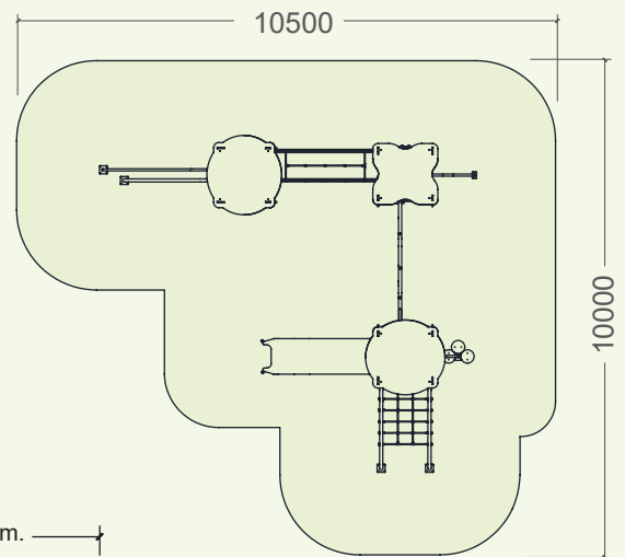
COMPLEJO DE TREPA 3 TORRES (CON TOBOGÁN PE) CLIMBING COMBINATION WITH 3 TOWERS (WITH PE SLIDE) COMBINAISON À GRIMPER AVEC 3 TOURS (AVEC TOBOGGAN PE)
